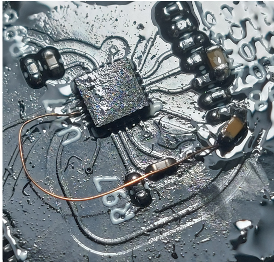
(a) Firul ce leaga unul dintre LDO-uri de un condensator. TODO BETTER PICTURE (b) Firul USB RX-TX TX-RX. TODO BETTER PICTURE
